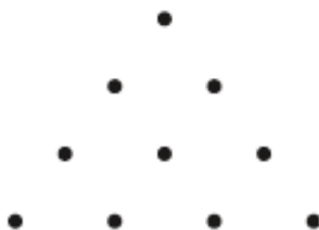
Слика 13: Тетрактис
