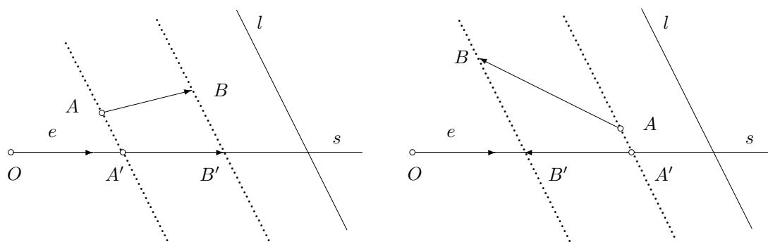
Slika 9. Paralelna projekcija
