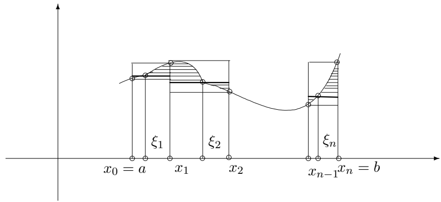
Slika 1. Rimanov integral
