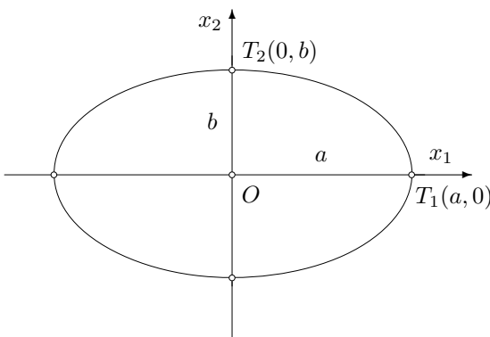
Slika 40. Elipsa
