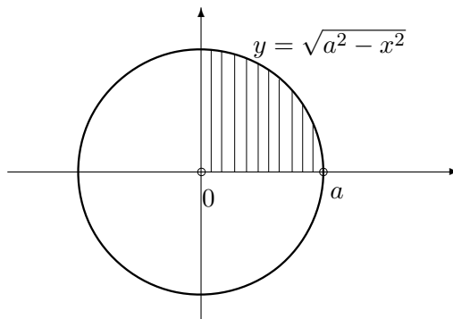
Slika 5. Geometrijski smisao
