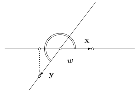
Slika 13. Skalarni proizvod
