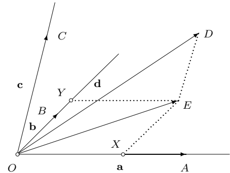
Slika 10. Razlaganje vektora u prostoru
