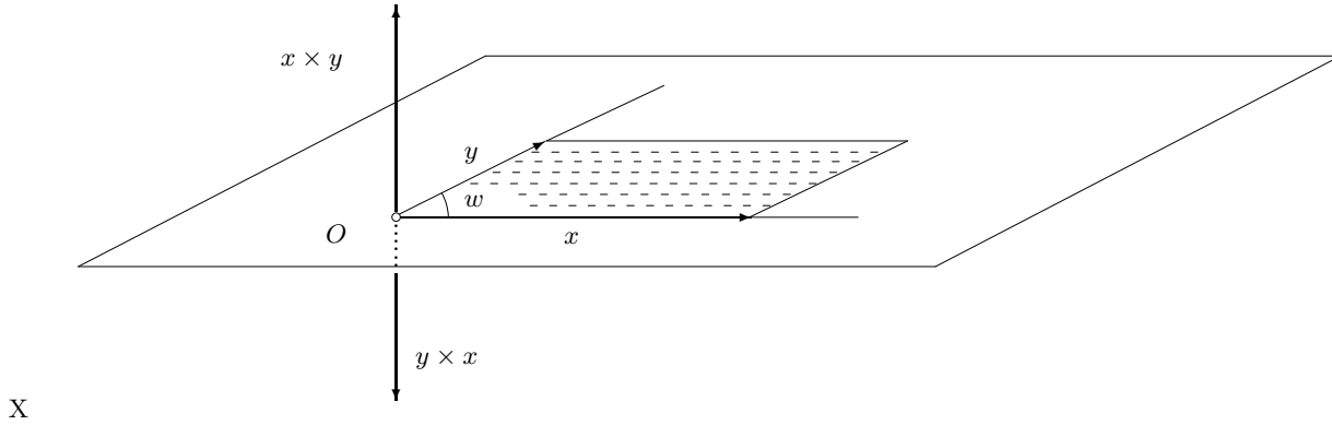
Slika 19. Vektorski proizvod
