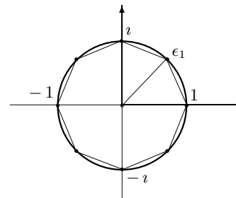
X Slika 2. n -ti koreni iz 1 ( n = 8 )
