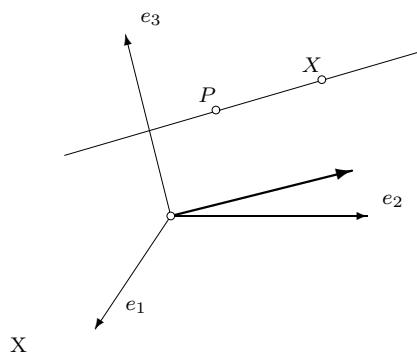
Slika 30. Prava
