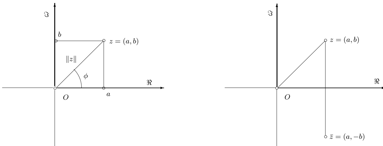
Dekartov i polarni oblik kompleksnog broja
