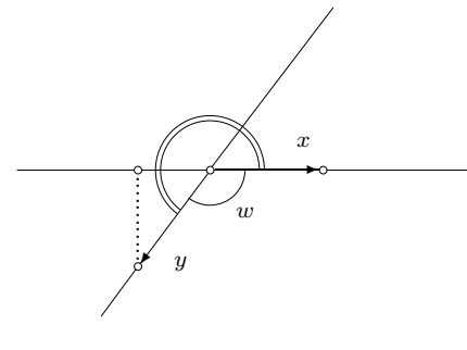
Slika 16. Skalarni proizvod
