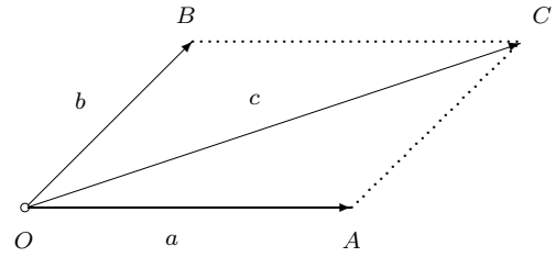
Slika 5. Zakon paralelograma
