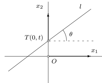
X Slika 24. Eksplicitni oblik jednačine prave
