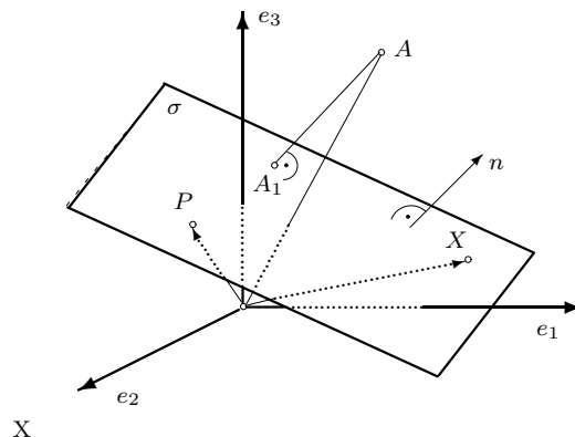
Slika 29. Ravan
