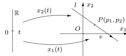
X Slika 25. Parametarska jednačine prave
