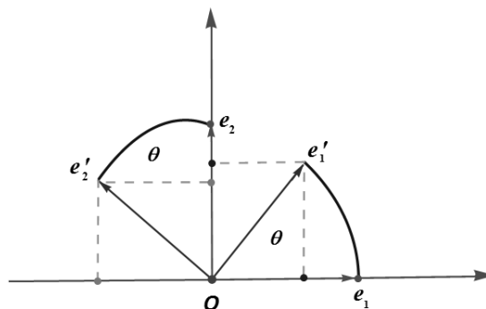
Slika 1. Rotacija u ravni
