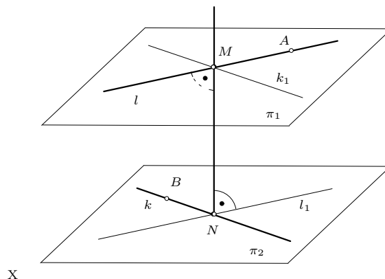
Slika 32. Zajednička normala
