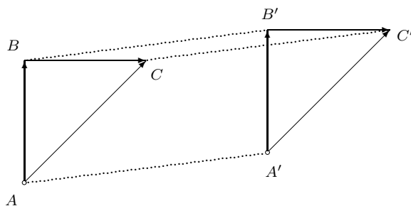
Slika 4. Nezavisnost sabiranja vektora od predstavnika
