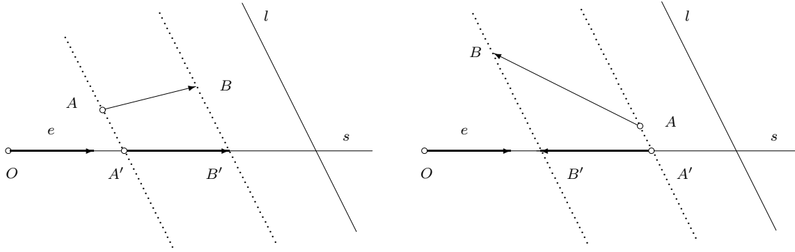
Slika 12. Paralelna vektor i skalar-projeksija
