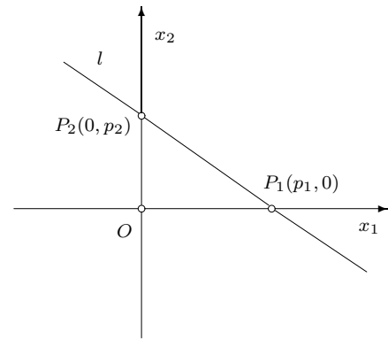
X Slika 23. Segmentni oblik jednačine prave
