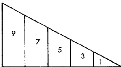
Слика 8: Пређени пут по равномерно убрзаном кретању је пропорционалан квадрату протеклог времена
