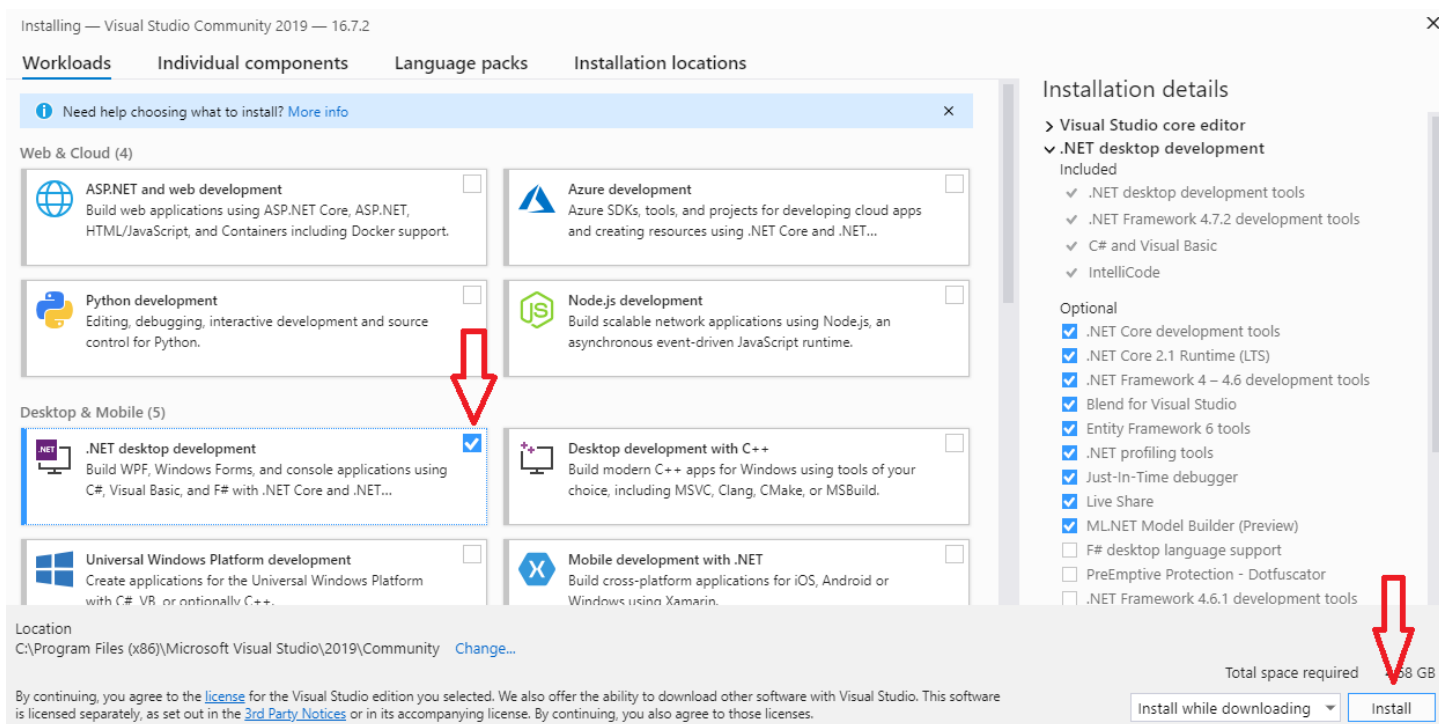
Slika 8. Pokretanje instalacije
