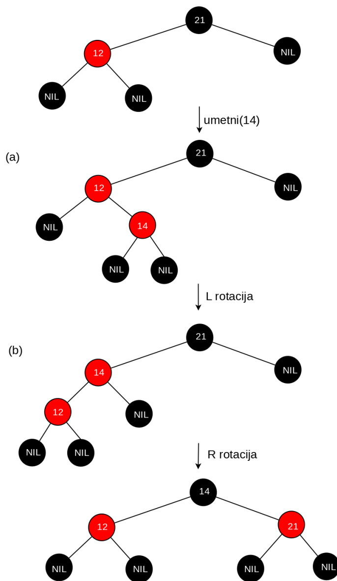
Slika 4: Primer umetanja elementa u crveno-crno drvo kada je roditelj novog čvora crven, a stric novog čvora crn.
