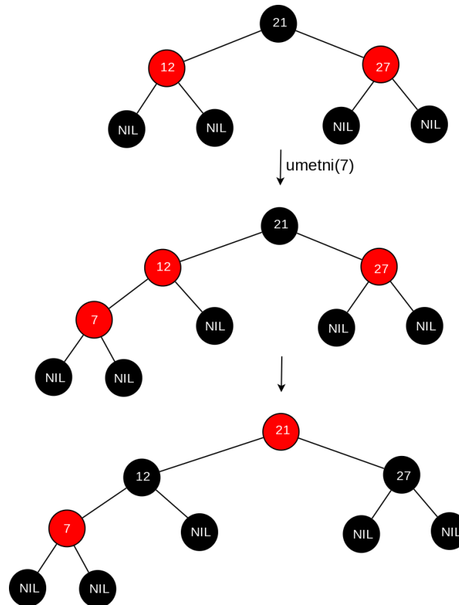
Slika 3: Primer umetanja elementa u crveno-crno drvo kada su i roditelj i stric novog čvora crveni.
