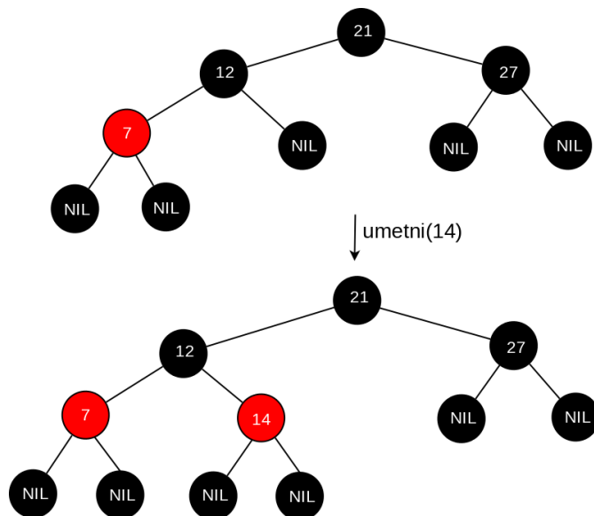
Slika 2: Primer umetanja elementa sa vrednošću 14 u crveno-crno drvo kojim se ne narušava nijedna od invarijanti crveno-crnog drveta.
