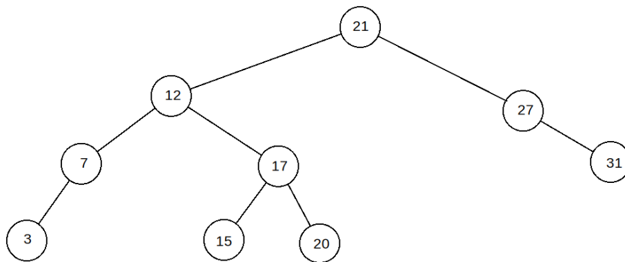
Slika 6: AVL drvo.
