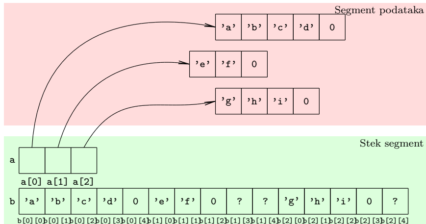
Slika 10.1: Niz pokazivača i dvodimenzioni niz u memoriji
