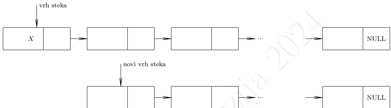
Slika 6.6: Ilustracija osnovnih operacija nad stekom implementiranim korišćenjem povezane liste
