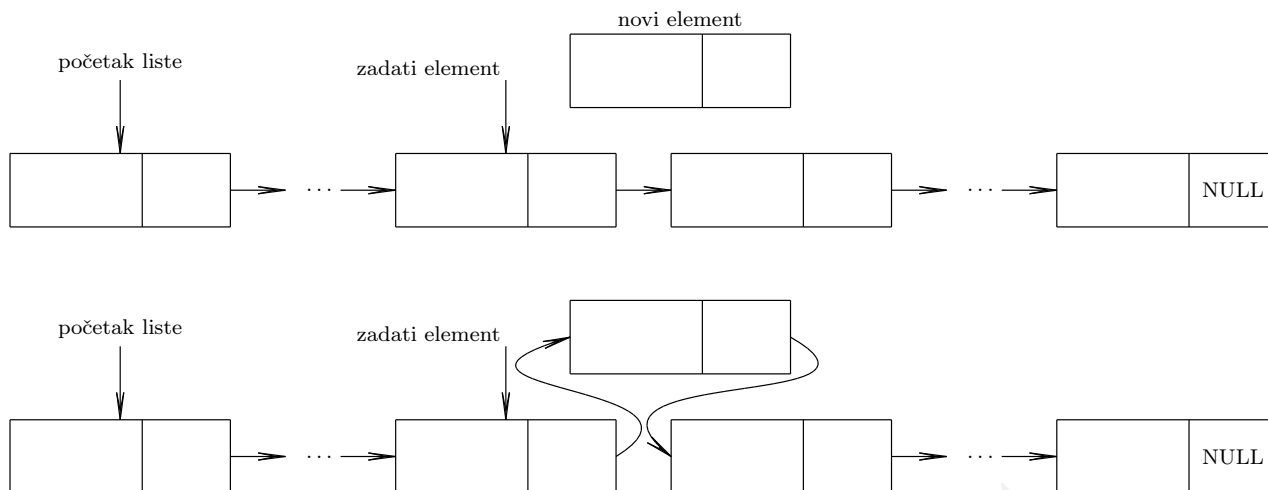
Slika 6.3: Ilustracija ubacivanja elementa u povezanu listu iza zadanog elementa
