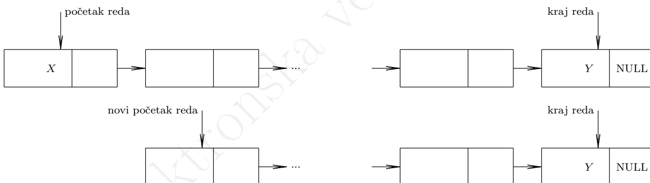
Slika 6.7: Ilustracija osnovnih operacija nad redom implementiranim kao povezana lista
