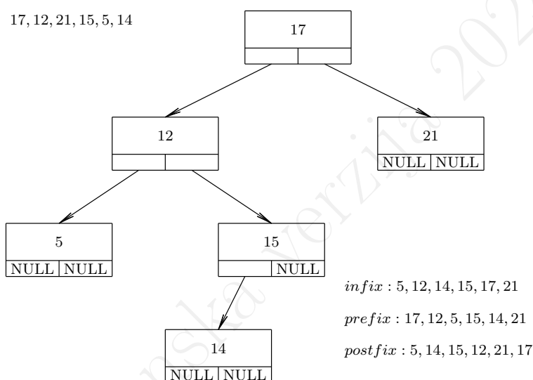
Slika 6.9: Uređeno binarno stablo
