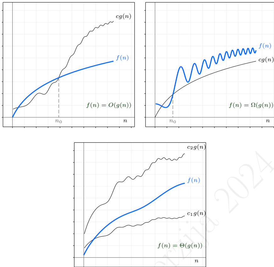
Slika 3.4: Ilustracija pojmova „veliko o“, „veliko omega“ i „veliko teta“
