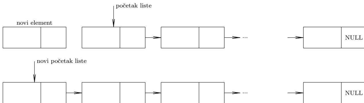
Slika 6.2: Ilustracija dodavanja elementa na početak povezanoj listi
