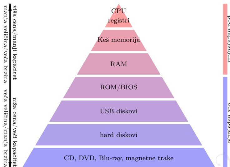
Slika 1.10: Memorijska hijerarhija
