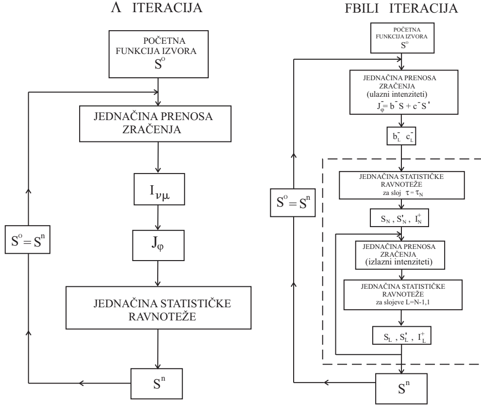
SI.1. Šema klasične \Lambda iteracije i FBILI iteracije
