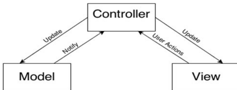
Slika 3: MVC arhitektura
