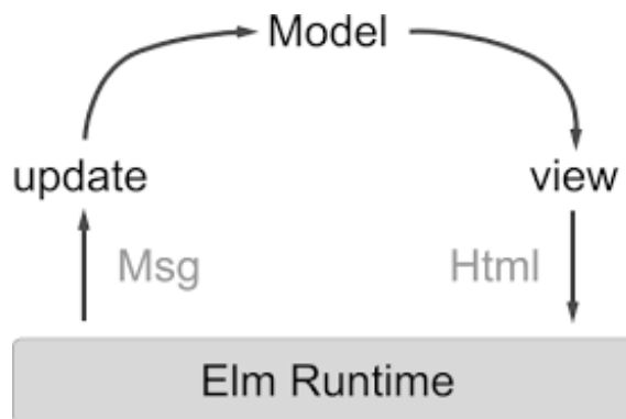
Slika 3.5: Arhitektura Elm [35]
