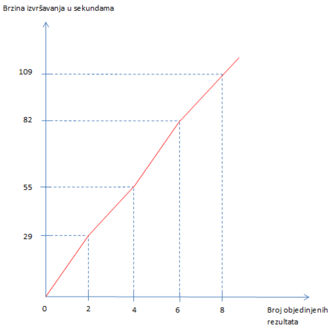
Slika 4.14: Dijagram izvršavanja algoritma DSK
