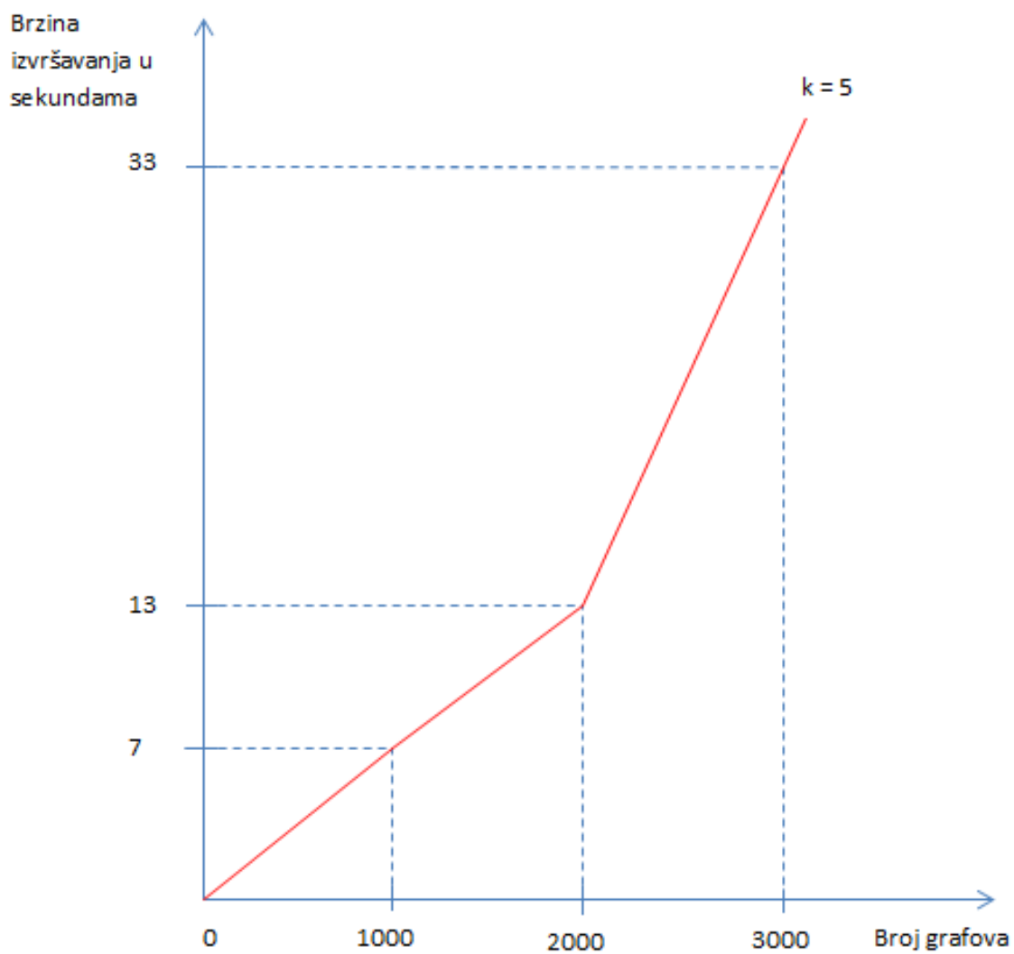
Slika 4.16: Dijagram izvršavanja algoritma AllEulerianCycles
