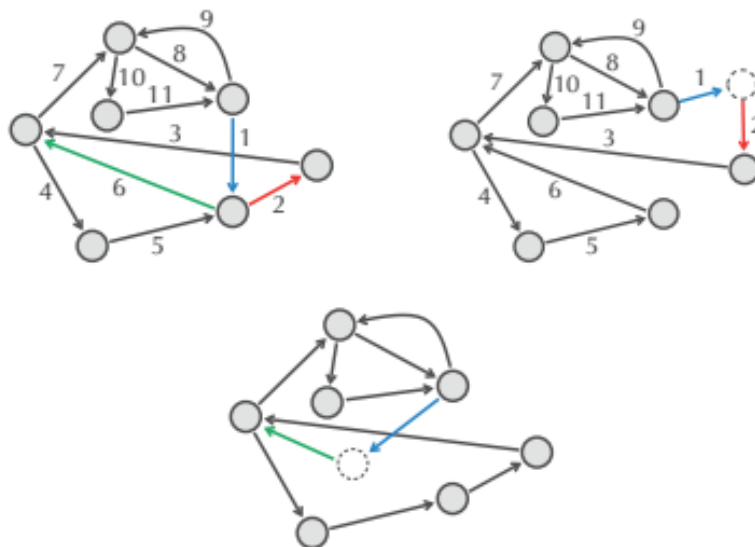
Slika 4.6: Primer kreiranja obilaznog grafa [5]
