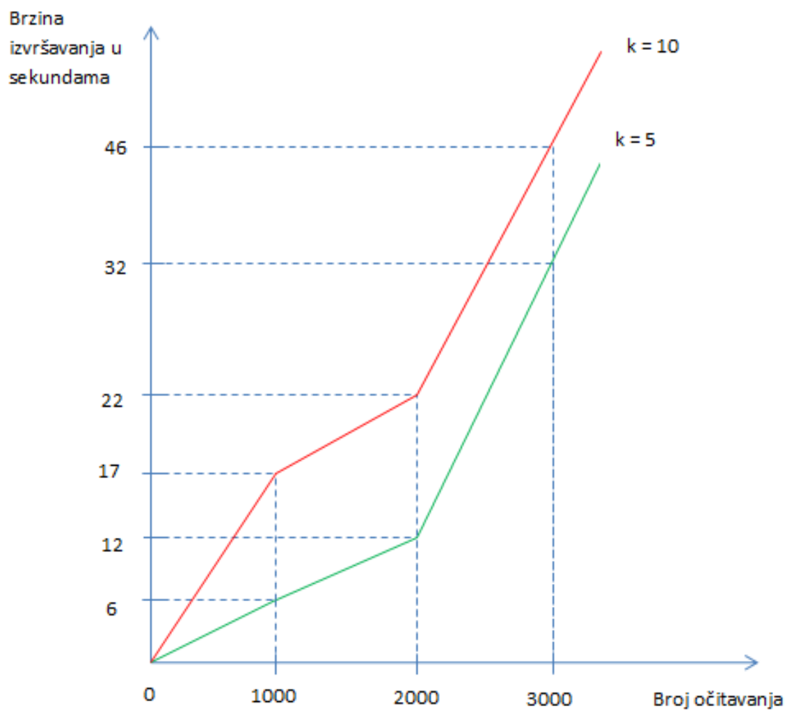
Slika 4.15: Dijagram izvršavanja algoritma DeBruijnGraph
