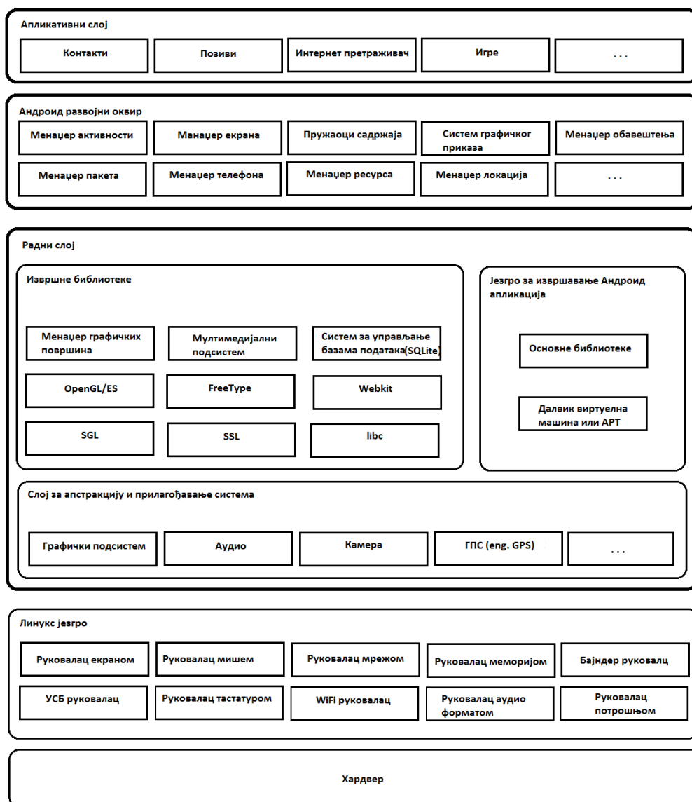
Слика 2.2: Архитектура Андроид оперативног система
