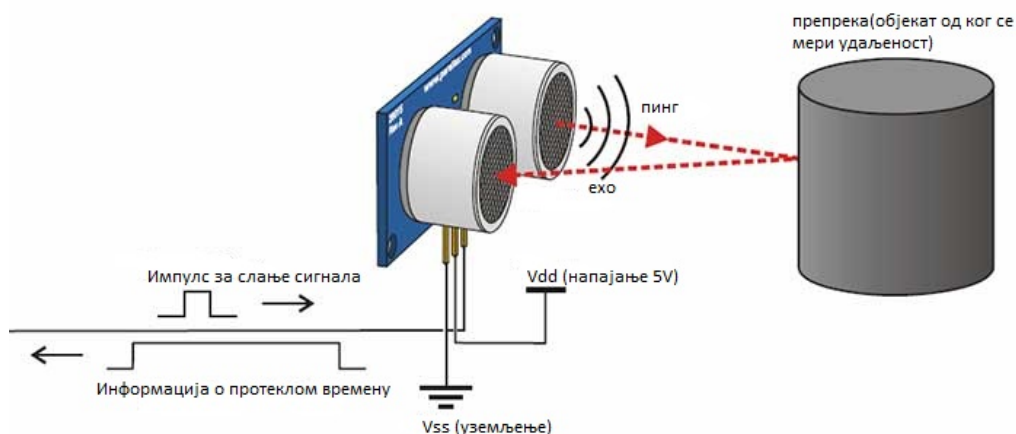
Слика 3.4: Принцип рада и изглед сензора удаљености
