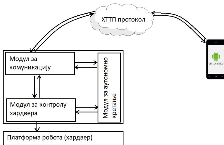
Слика 5.5: Сликвит приказ модула апликације на Разберију и њихове сарадње
