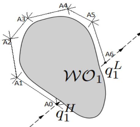
Слика 4.4: Начин рада БАГ2 алгоритма на роботу
