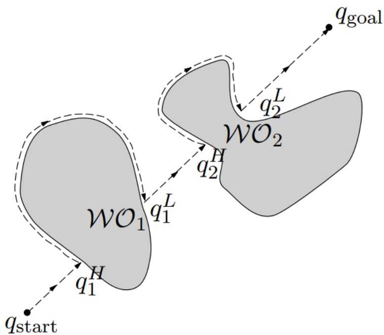
Слика 4.2: Начин рада алгорита БАГ2
