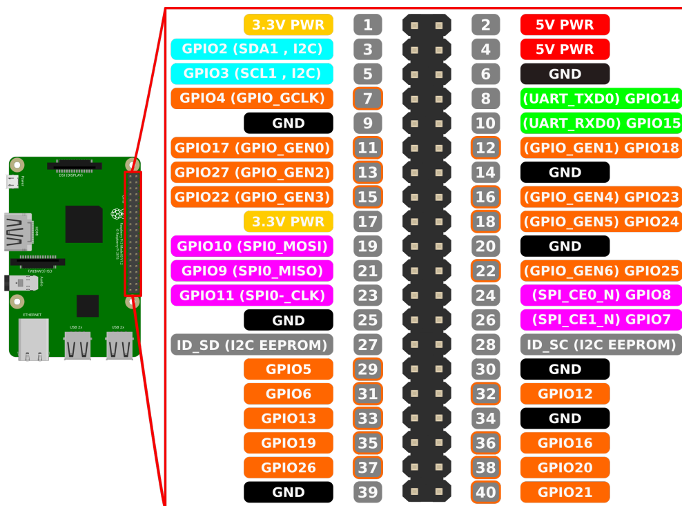
Слика 3.1: Називи и распоред GPIO пинова на Разбери Пај 3
