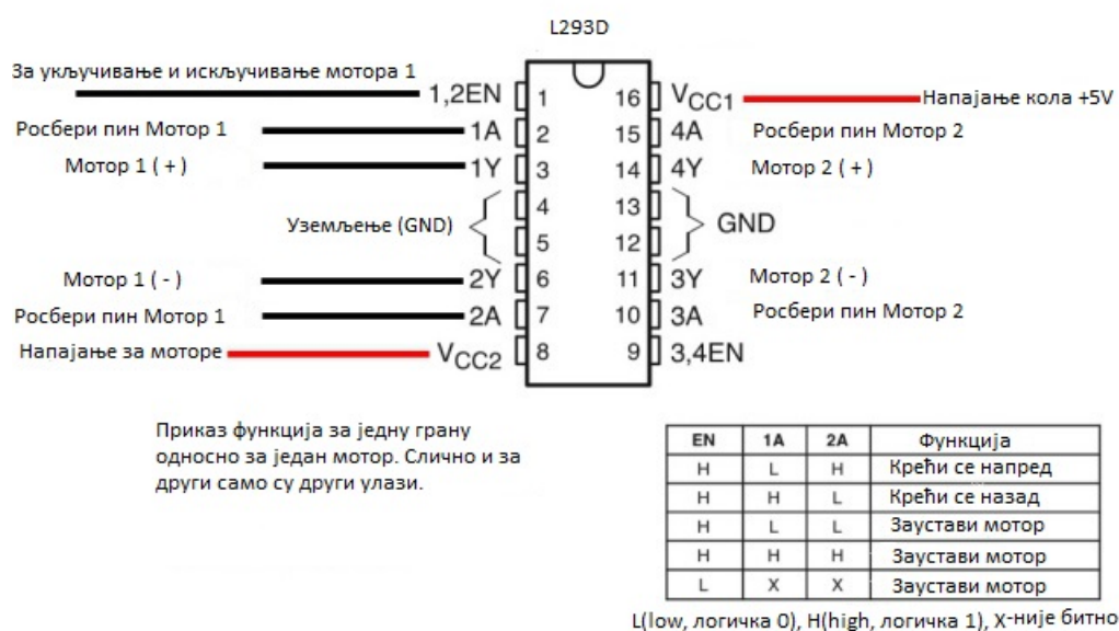
Слика 3.3: Мотор контролер L293D
