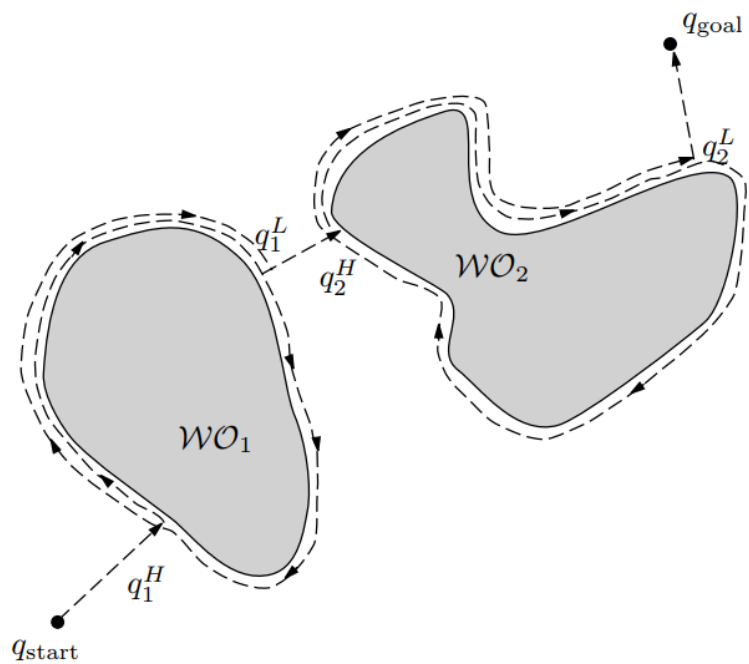
Слика 4.1: Начин рада алгорита БАГ1
