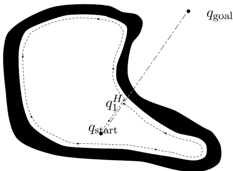
Слика 4.3: Детекција случаја када не постоји пут до циља
