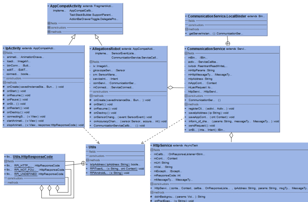
Слика 5.4: Дијаграм класа Андроид апликације
