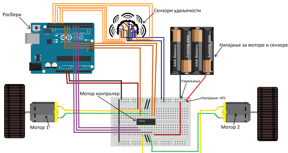
Слика 3.5: Шема за повезивање Разберија са платформом и сензорима
