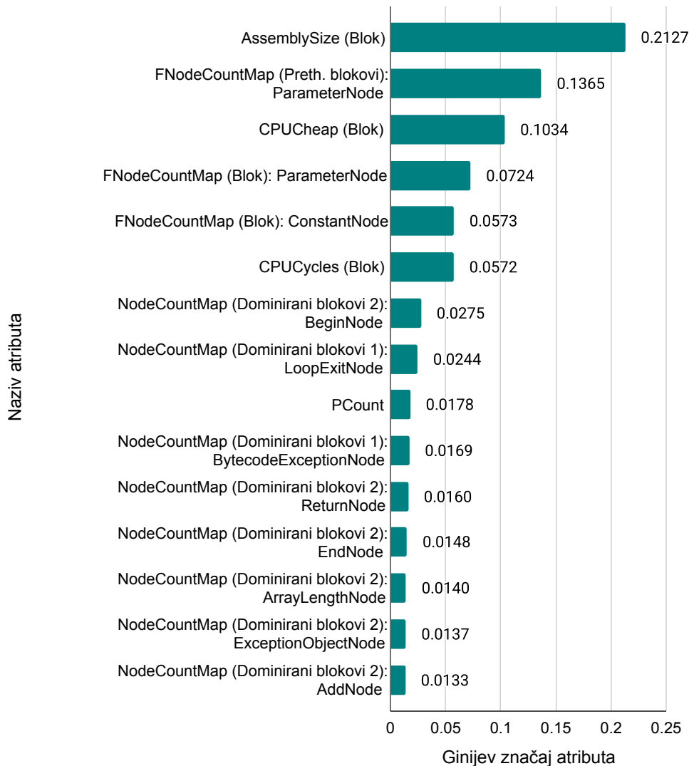
Slika 6.1: Atributi kojima se opisuju naredbe grananja sortirani na osnovu Ginijevog značaja i obučenog modela stabla odlučivanja. Za attribute predstavljene rečnicima NodeCountMap i FNodeCountMap dat je i konkretan naziv čvora odnosno ključa rečnika.
