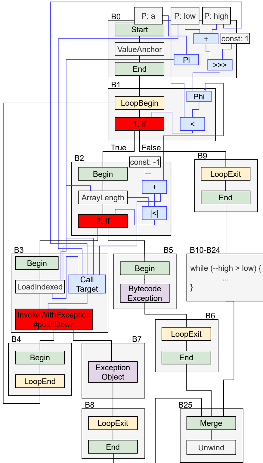
Slika 4.2: Gaal IR graf i graf kontrole toka koji odgovaraju for petlji funkcije heapSort (funkcija je prikazana na listingu 2)
