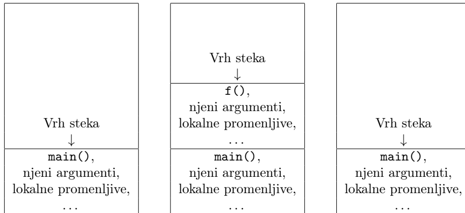
Slika 10.1: Organizacija steka i ilustracija izvršavanja funkcije. Levo: tokom izvršavanja funkcije main() . Sredina: tokom izvršavanja funkcije f() neposredno pozvane iz funkcije main() . Desno: nakon povratka iz funkcije f() nazad u funkciju main() .
